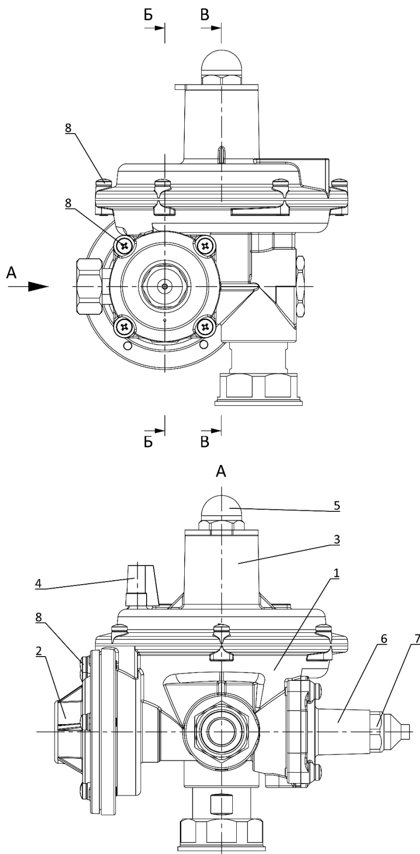
Рисунок 1 – Устройство регулятора давления «РЕД-2-20х32Р-...».
