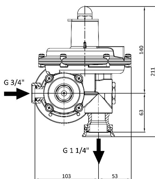
Исполнение регулятора давления "РЕД-2-20x32P-..."
